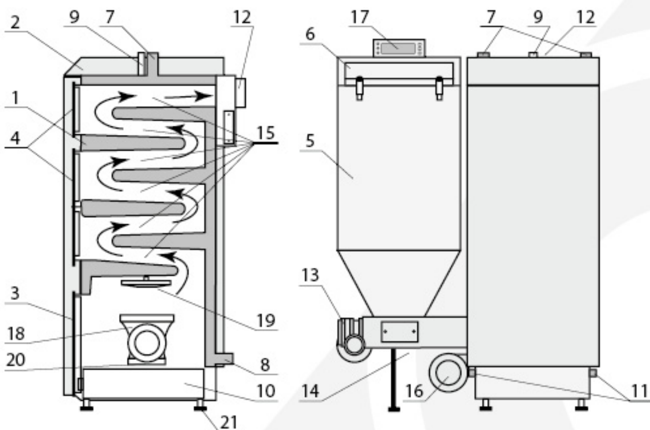
Kotły wodne typu TORET
